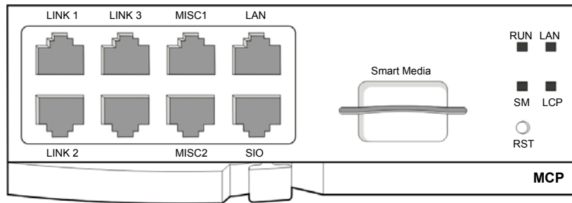
Рис. 2.2 Плата МСР - вид спереди
